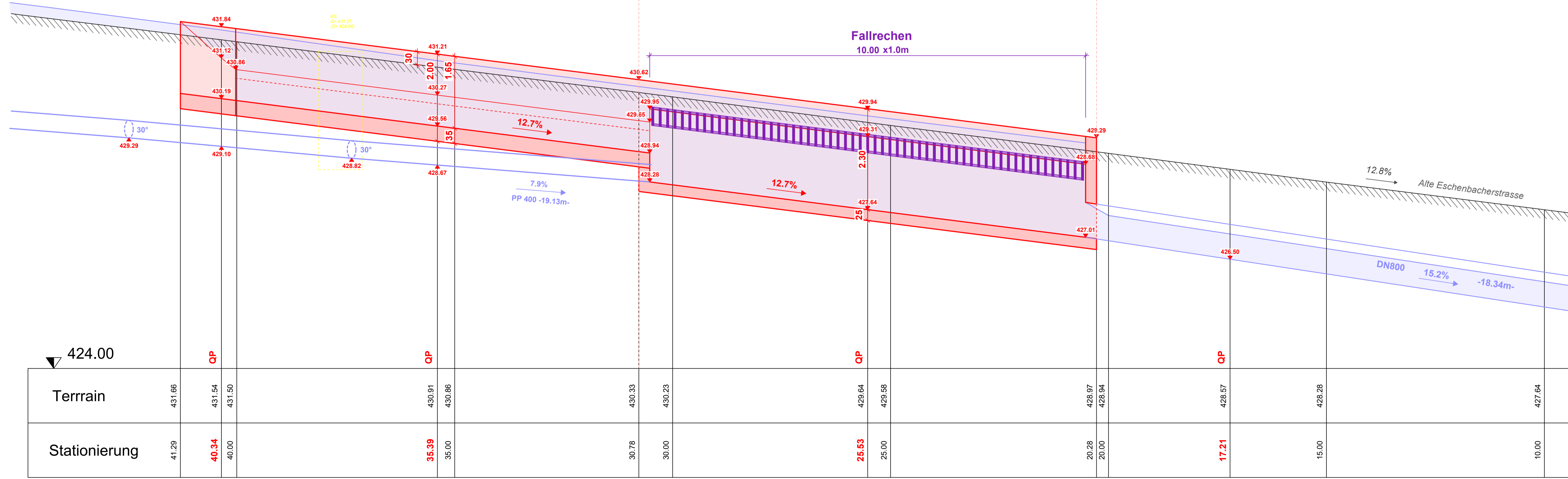
Längsschnitt 1:50
